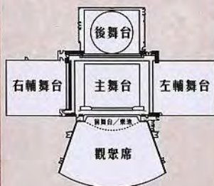
葵青劇院舞台平面圖
