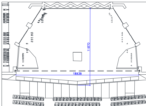
反音板設計
