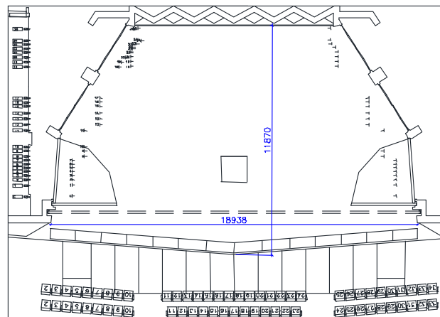
反音板設計
