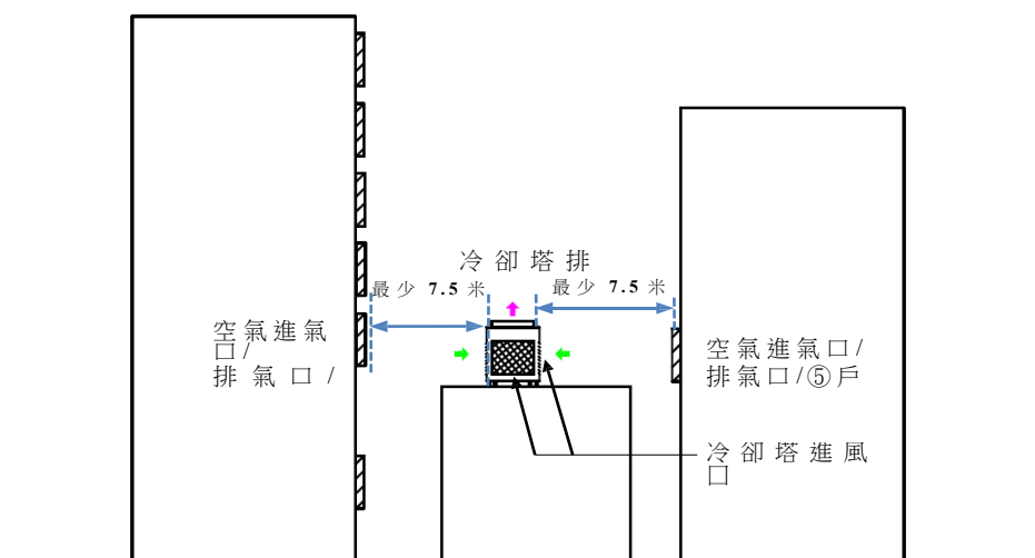
圖 3: 冷卻塔安裝於屋頂及被周邊建築物包圍，須與周邊建築物的空氣進氣口、排氣口、可開啟⑤戶及公眾通道水平相距至少 7.5 米。
