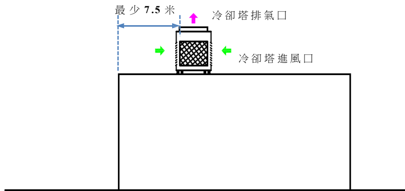
圖 1: 冷卻塔安裝於屋頂並與附近的空氣進氣口、排氣口、可開啟⑤戶及公眾通道水平相距至少 7.5 米。
