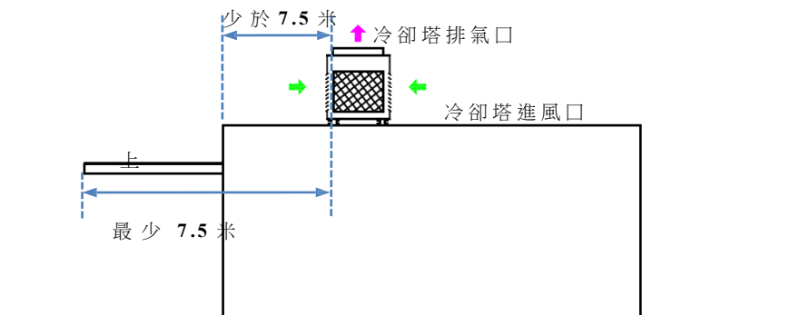
圖 2: 冷卻塔安裝於屋頂並與附近的空氣進氣口、排氣口、可開啟⑤戶及公眾通道水平相距至少 7.5 米。
