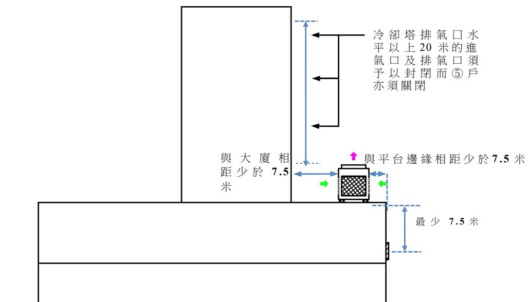
圖 6: 冷卻塔安裝於平台(與平台邊緣及平台上大廈水平相距少於 7.5 米)須與垂直建築面上的進氣口、排氣口和可開啟 ⑤ 戶垂直相距最少 7.5 米(冷卻塔水平以下)或 20 米(冷卻塔水平以上)。冷卻塔 7.5 米水平範圍內不可讓公眾進入。
