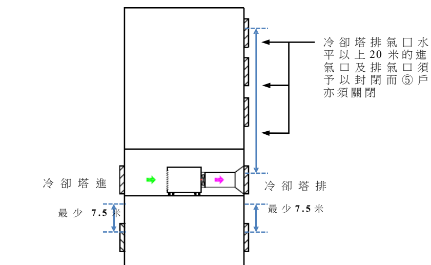
圖 4: 冷卻塔安裝於室內須與垂直建築面上的進氣口、排氣口和可開啟⑤戶垂直相距最少 7.5 米（冷卻塔水平以下）或 20 米（冷卻塔水平以上）。
