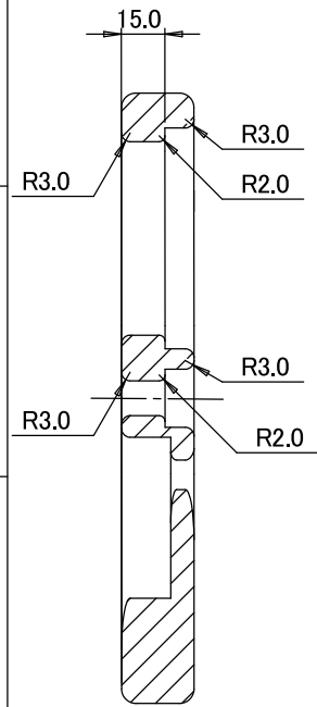
SECTION A-A
